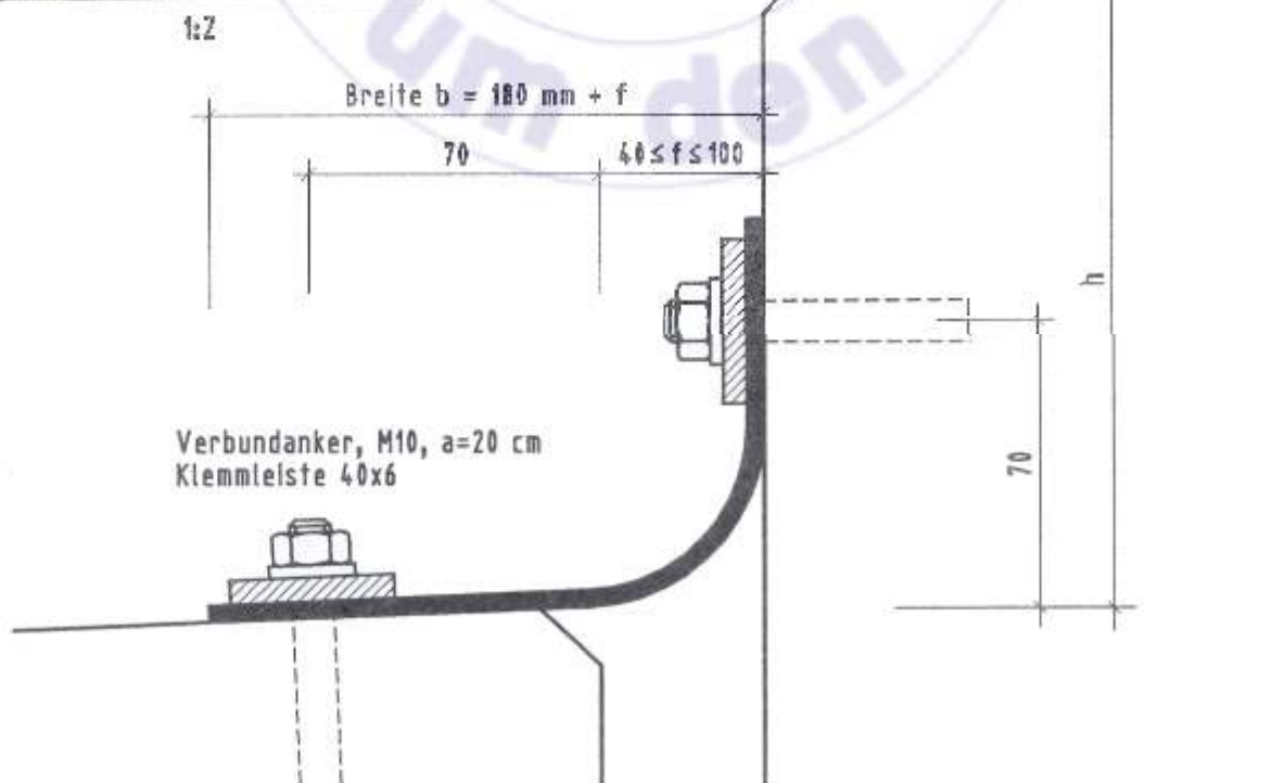
Bild 2: h > 150 mm
