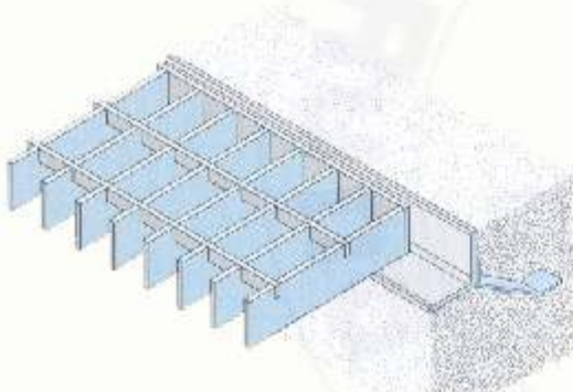
Rahmen für herausnehmbare Roste
