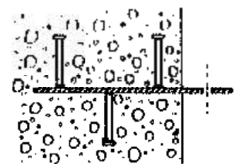
FLANSCH KOPFBOLZEN AUF FLACHSTAHL GESCHWEISST
