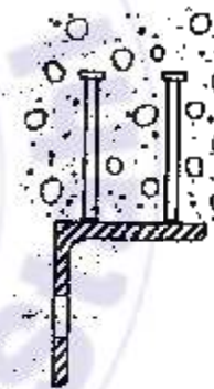
GESTUFTE ECKAUSBILDUNG AUF SCHWEISSEN ZWEIER KOPFBOLZEN AUF EIN Z-PROFIL
