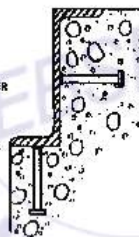
GESTUFTE ECKAUSBILDUNG AUF SCHWEISSEN ZWEIER KOPFBOLZEN AUF EIN Z-PROFIL
