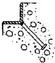
GESTUFTE ECKAUSBILDUNG AUF DIE ECKE EINES WINKELS AUFGESCHWEISSTER KOPFBOLZEN
