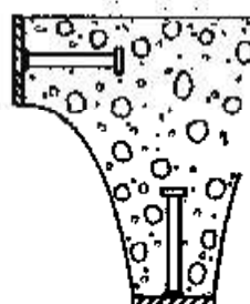
GEBÄLDE- AUSBILDUNG AUF SCHWEISSEN VON KOPFBOLZEN AUF FLACHEISEN
