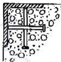
ECKAUSBILDUNG ZWEI AUF EINANDER IN DIE ECKE EINES WINKELS GESCHWEISSTE KOPFBOLZEN
