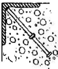
ECKAUSBILDUNG ZWEI AUF EINANDER IN DIE ECKE EINES WINKELS GESCHWEISSTE KOPFBOLZEN
